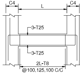
BEAM(350x400)
